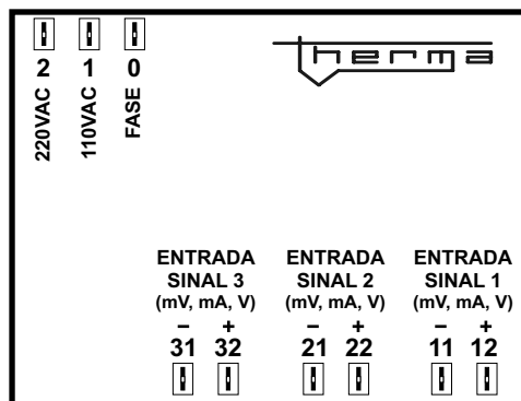
INDICADOR TH 2063-2
