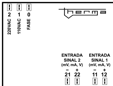
INDICADOR TH 2062-2
